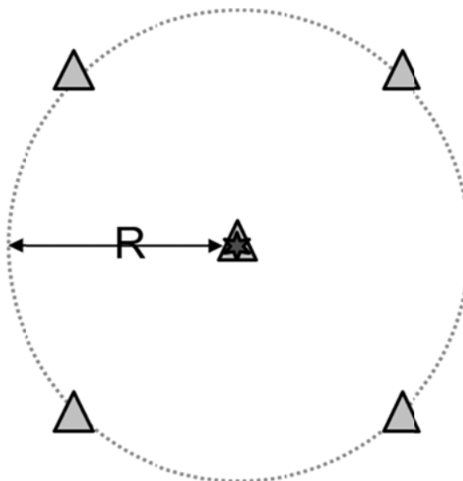
Abb. A1: Optimale Geometrie eines Stationsnetzwerkes mit 5 Stationen (Dreiecke) zur Lokalisierung von Erdbeben im Zentrum des Netzwerkes. Vereinfachende Annahmen: Homogenes Geschwindigkeitsmodell, gleiche Störsignalniveaus an den Stationsstandorten und geringe ( < 1 km) Ausdehnung der geotechnischen Anlage.
